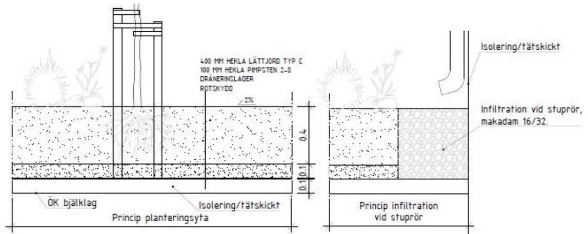
Figur 23. Förslag på uppbyggnaden av bjälklaget för att effektivt hantera dagvatten. Skiss från Sweco (2021).
