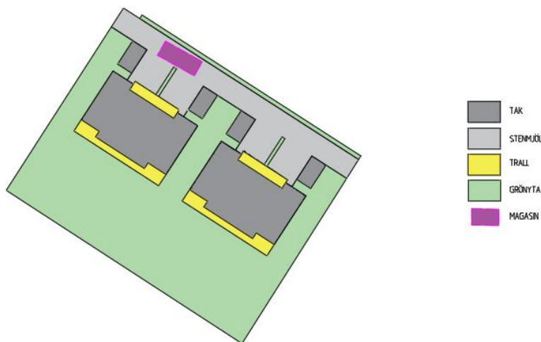
Figur 9. Framtida fastighet med dagvattenmagasin.
