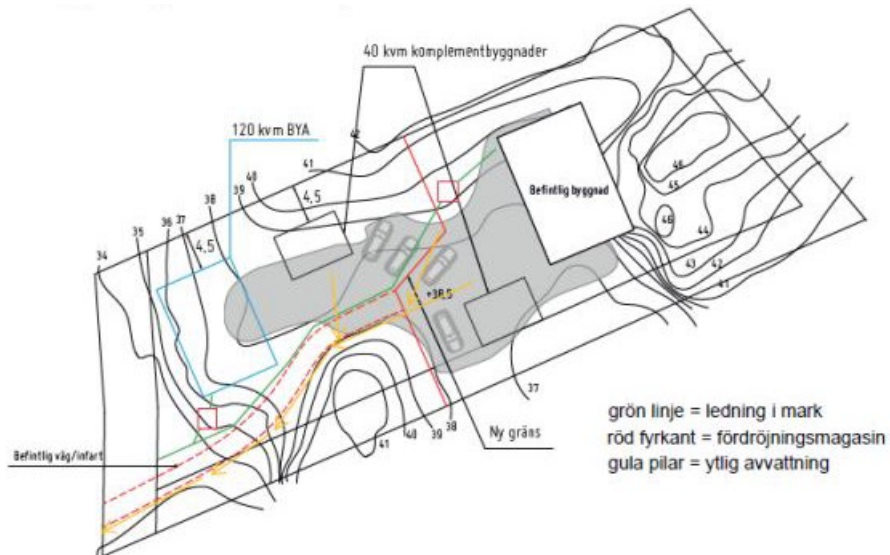
Figur 16. Gröna linjer markerar ledning i mark, röd fyrkant redogör förslag på placering av fördröjningsmagasin inom respektive fastighet. Gula pilar visar ytlig avvattning.
